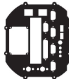
VT-EC11 · 5x DB9 · 1x DB25 · 2x USB · 2x PS2 · 2x RJ45 · 1x Floppy · 1x Power Supply · 3x Audio
