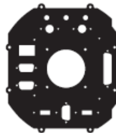
VT-EC10 · 3x DB9 · 1x DB15 · 2x USB · 2x DIN · 1x RJ45 · 3x 0.265" circular · 1x 2.125" fan
