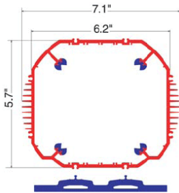
VersaTainer Dimensions
