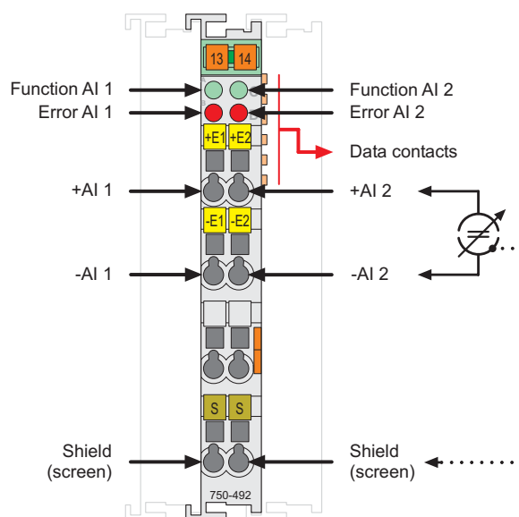
Fig. 2.1.1-1: 2-Channel Analog Input Module 4-20 mA
